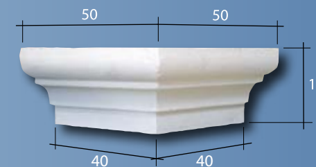
Angle sortant 30 Kg
