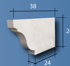
Bout fermé 5 Kg
