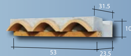
Génôise un entablement (non remplie 26 Kg, remplie 28 Kg)
