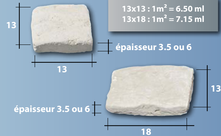
Joint de dilatation en pavés
