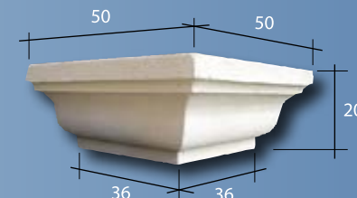
Angle sortant 34 Kg
