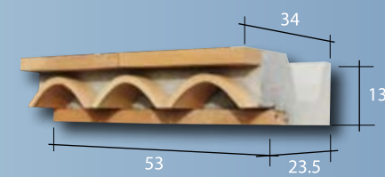
Génôise deux entablements (non remplie 29 Kg, remplie 31 Kg)
