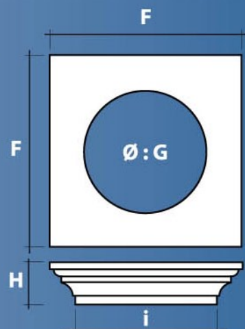
Chapiteau de 40 et 50 : 65/116 Kg
