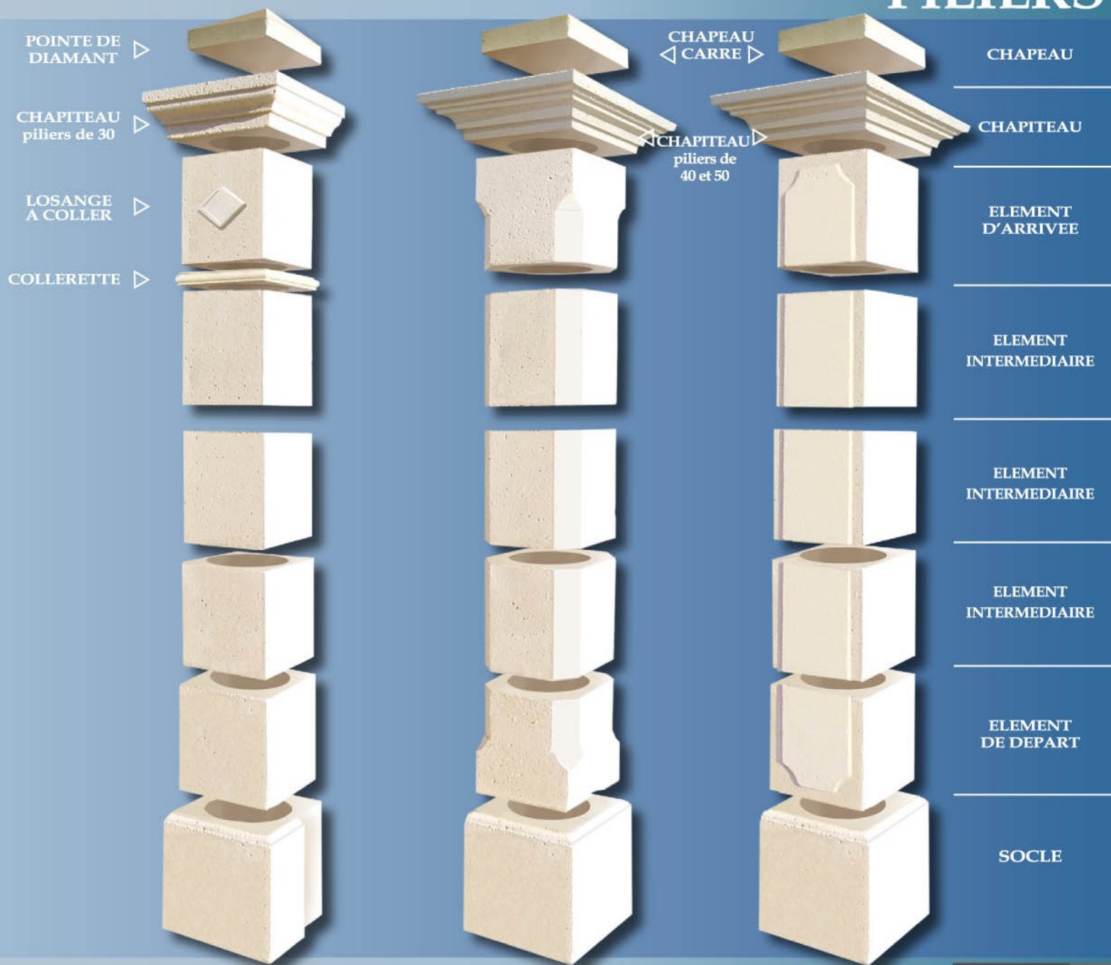
PILIER ANGLES VIFS
