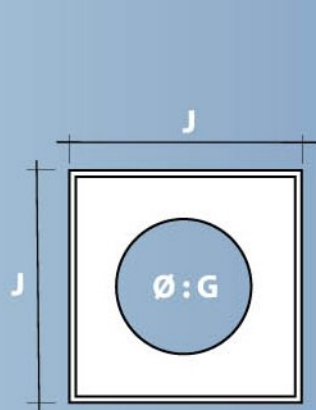
Chapeau carré de 30, 40 et 50 : 20/33/53 Kg
